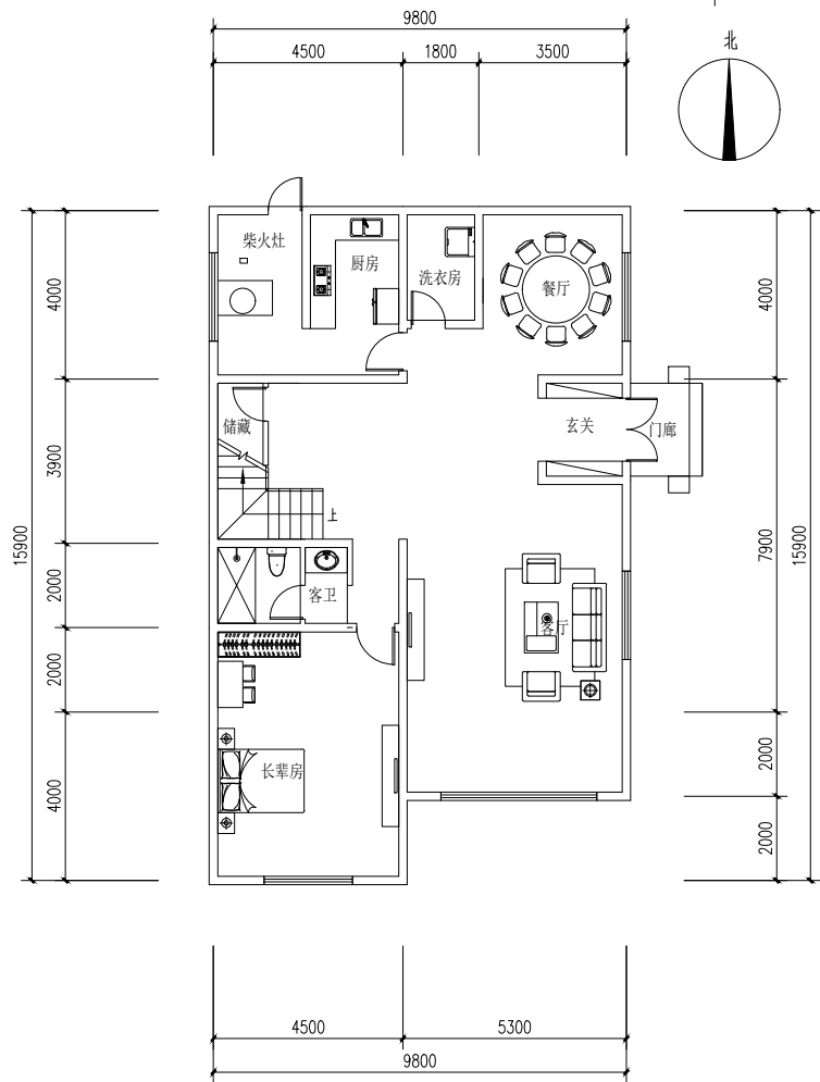
一层平面图 1:100
