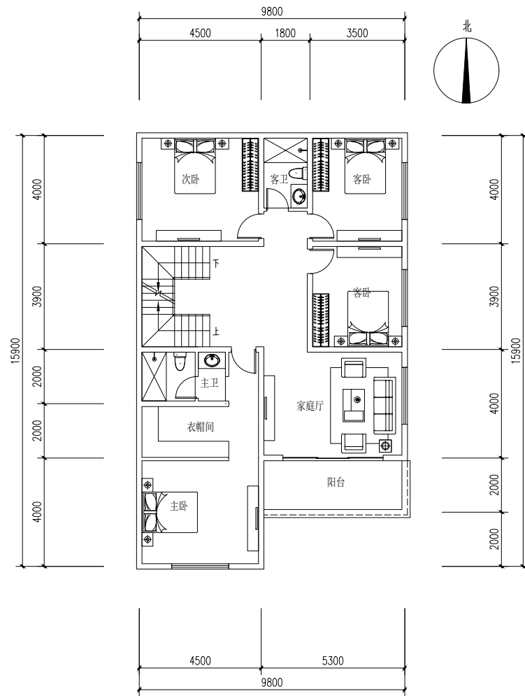
二层平面图 1:100
