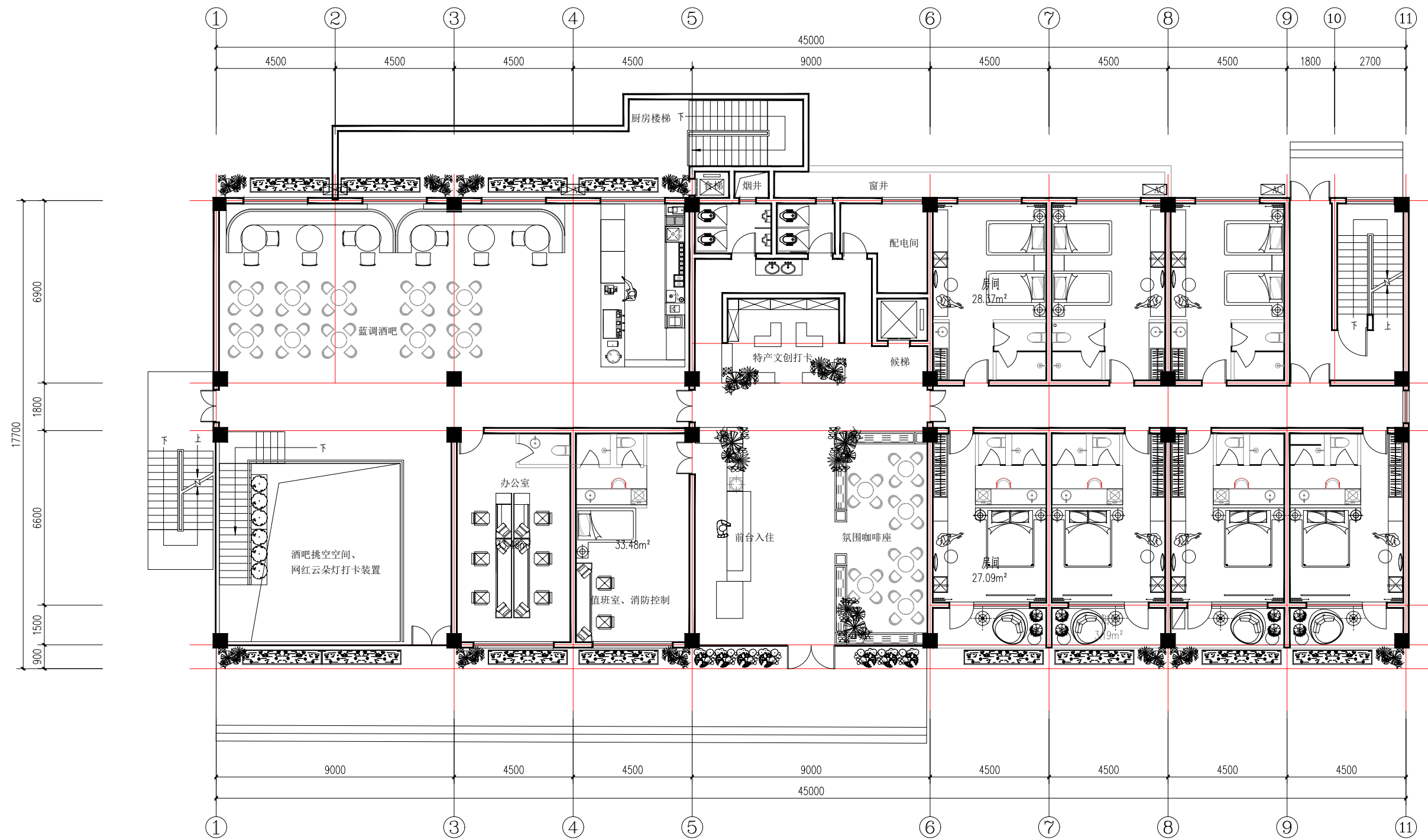
酒店民宿首层平面图 1:150
