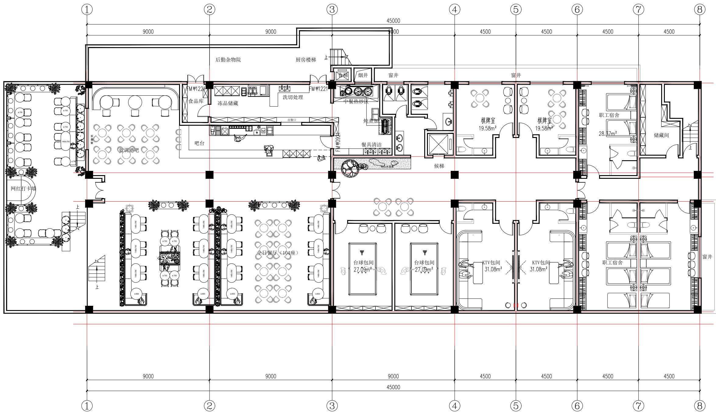
酒店民宿地下一层平面图 1:150
