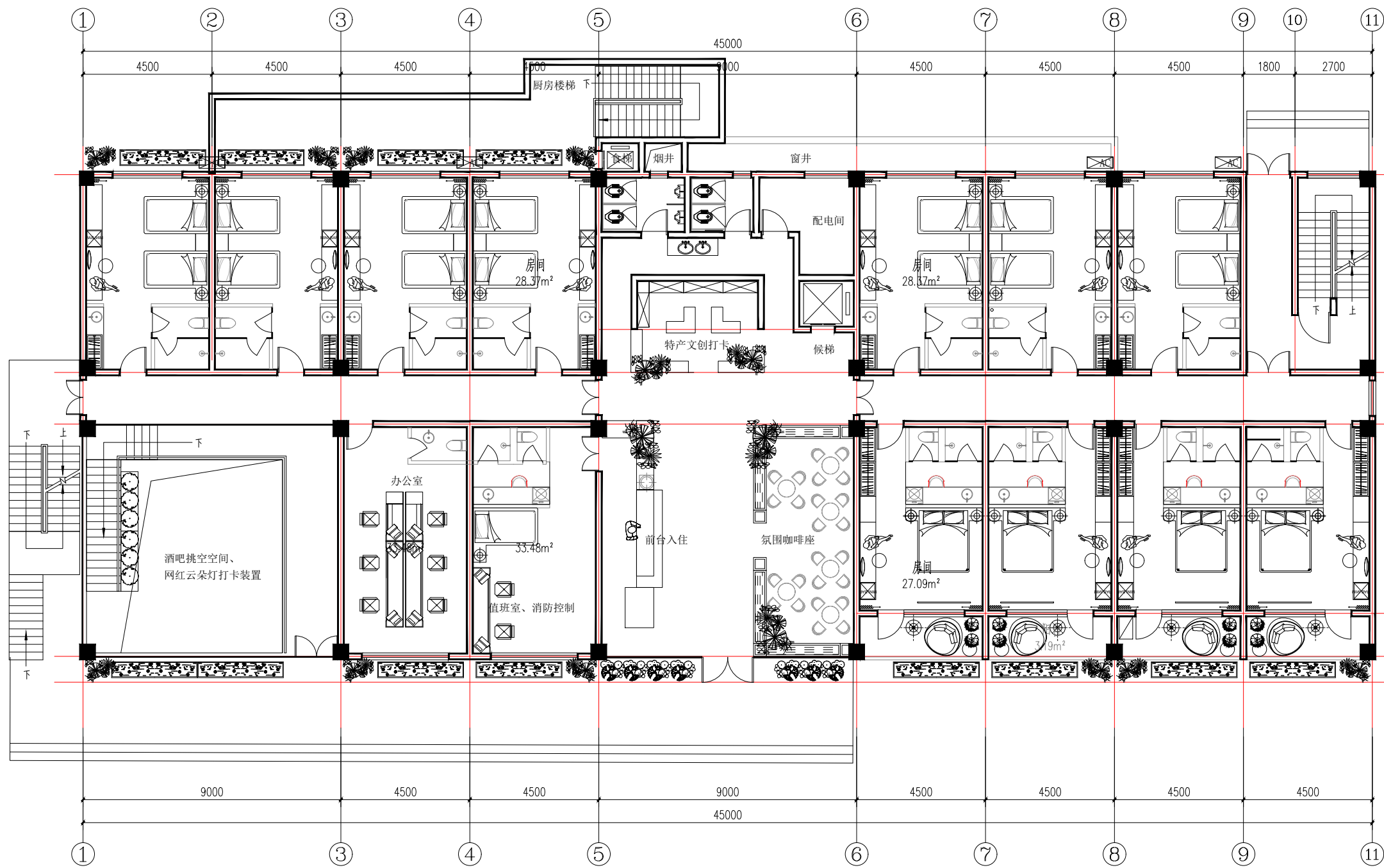
酒店民宿首层平面图 1:150
