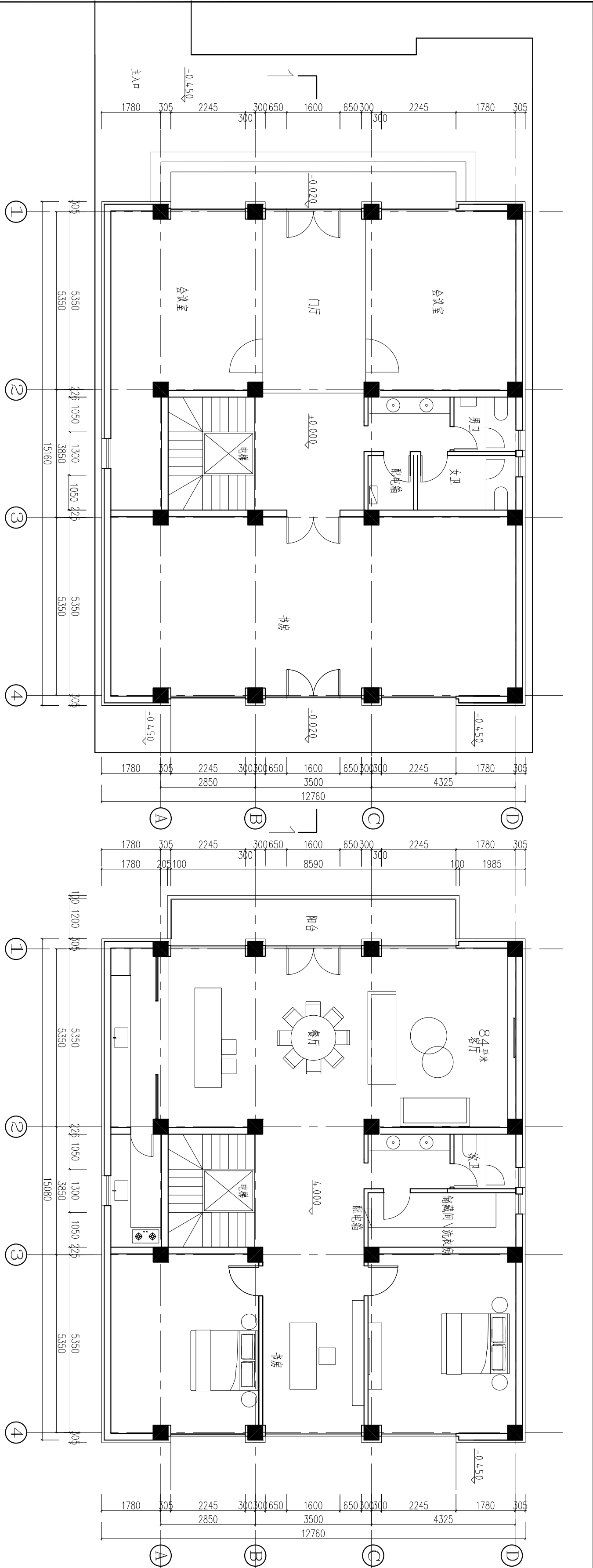
一层平面图
